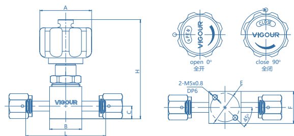
手动型 (带锁 VFS 内螺纹)
