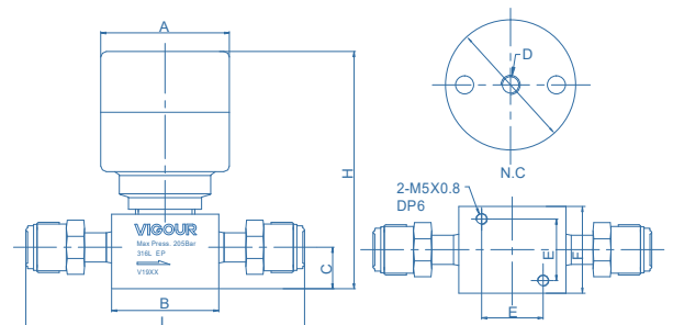
3/8, 1/2 气动型 (VFS 外螺纹 常闭)
