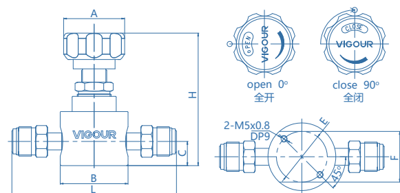
低压手动型 (VFS外螺纹)
