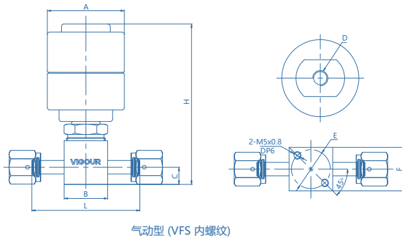
气动型 (常闭)
