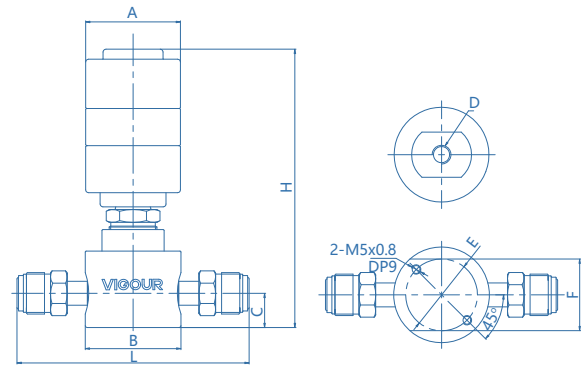
低压气动型 (VFS外螺纹)
