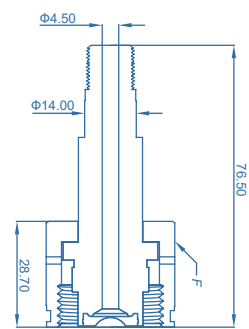
1/4"NPT(M)
