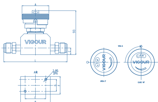
manual actuator
