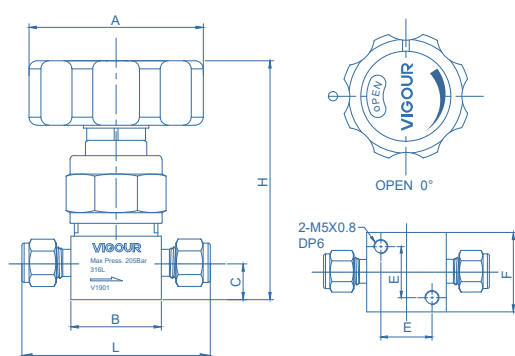
1/4, 3/8, 1/2 manual actuator
