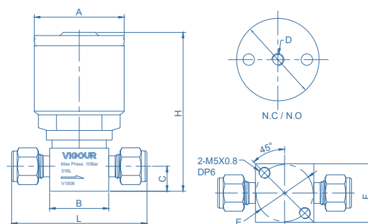
1/4 pneumatic actuator
