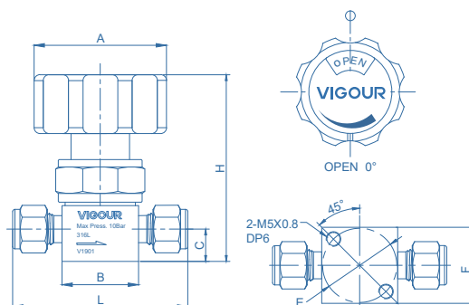
1/4, 3/8, 1/2 manual actuator
