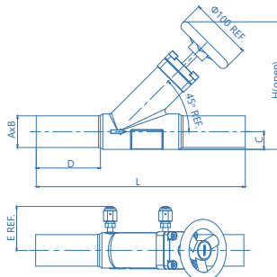
Manual Actuator 1.5~2"
