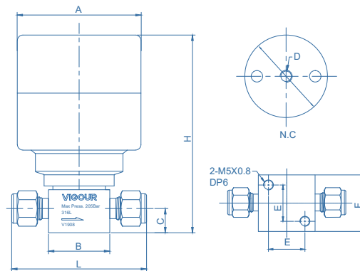
1/4, 3/8, 1/2 pneumatic actuator (N.C.)
