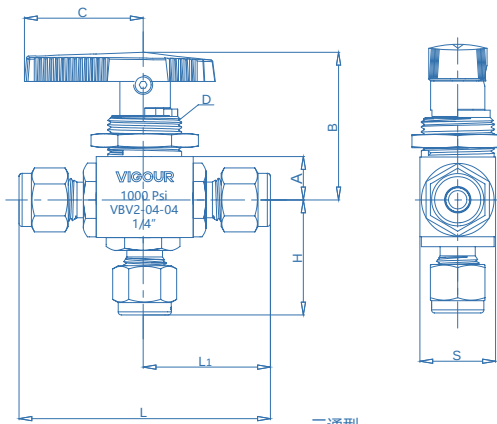
三通型
