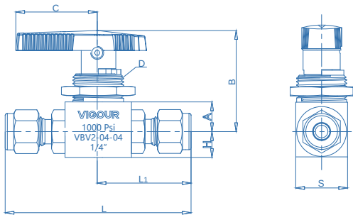
直通型
