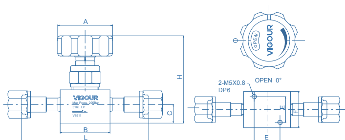
1/2 手动型 (VFS 内螺纹)
