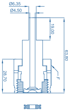
1/4" 焊接接管
