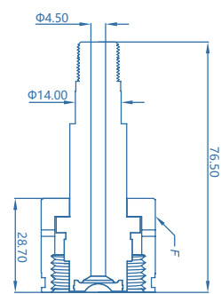
1/4"NPT(M)
