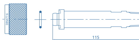
手拧螺帽和接杆 (举例: VCC-C-HNN-DIN477.6)
