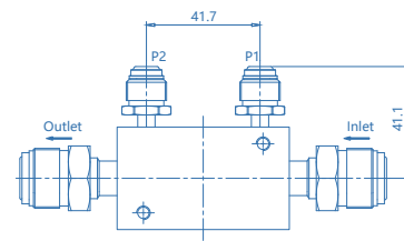
带吹扫口图示
