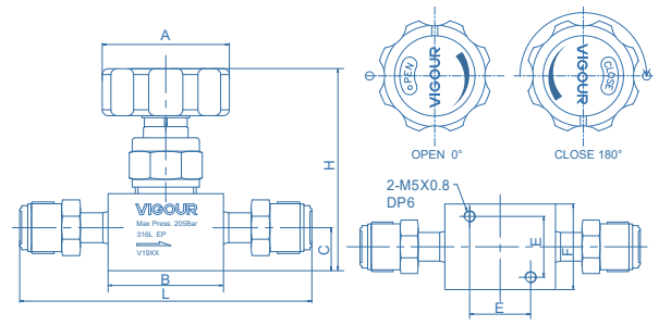
1/2 手动型 (VFS 外螺纹)
