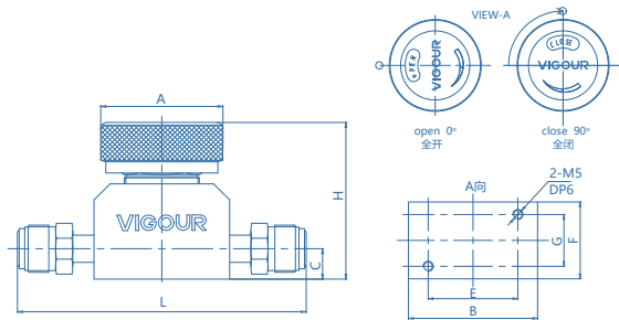
手动型 (VFS外螺纹)
