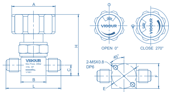
1/4手动型 (VFS 外螺纹)
