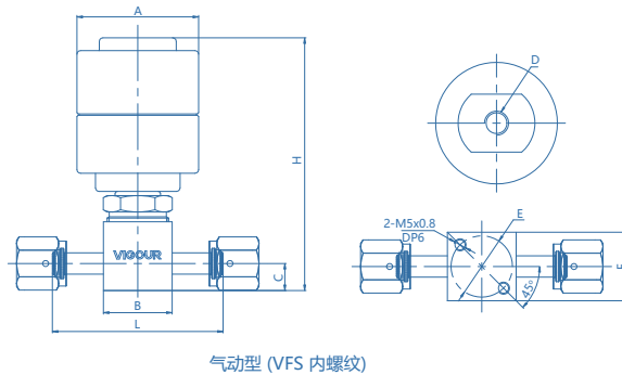
气动型 (常闭)
