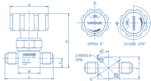
1/4, 1/2 手动型 (VFS 外螺纹)
