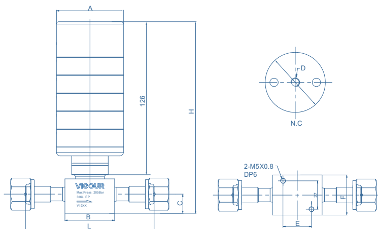
1/2 气动型 (VFS 内螺纹 常闭) HPC
